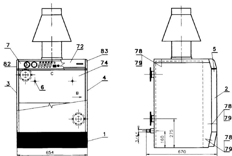
Umístění prvků kotle P 50 lux
