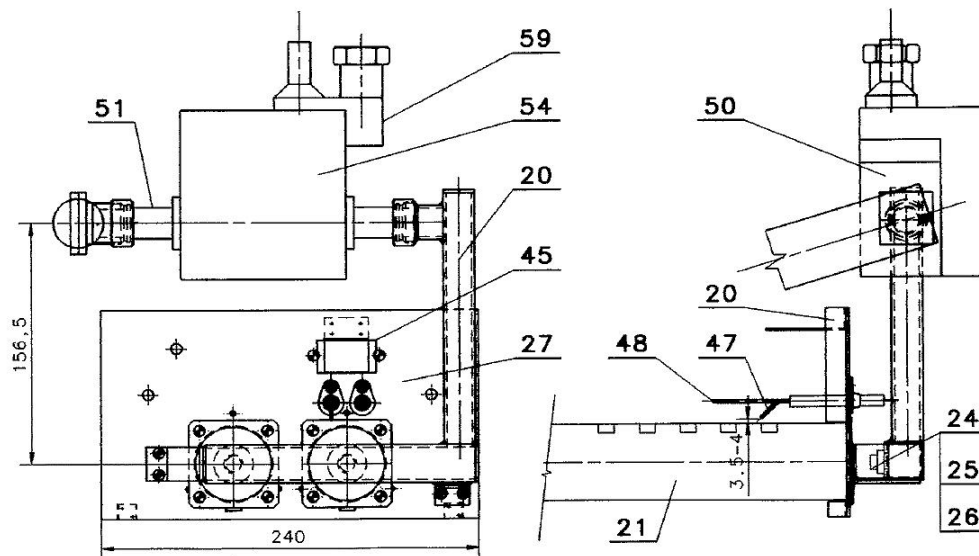
Hořák kotlů P lux 18-30 kW
