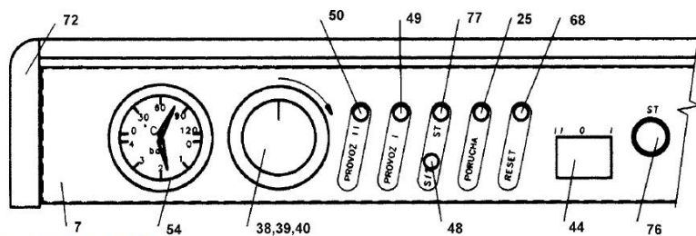
Ovládací panel kotle P 50 lux
