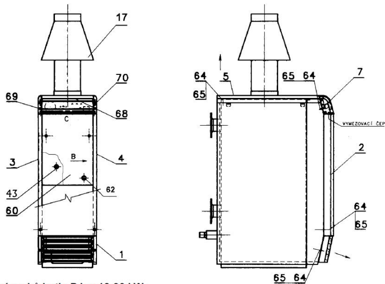
Umístění prvků kotle P lux 18-30 kW
